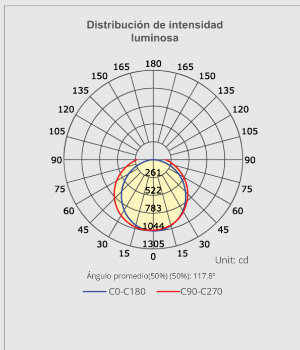
Gráfica del flujo lumínico de la luminaria DL-TPL003
